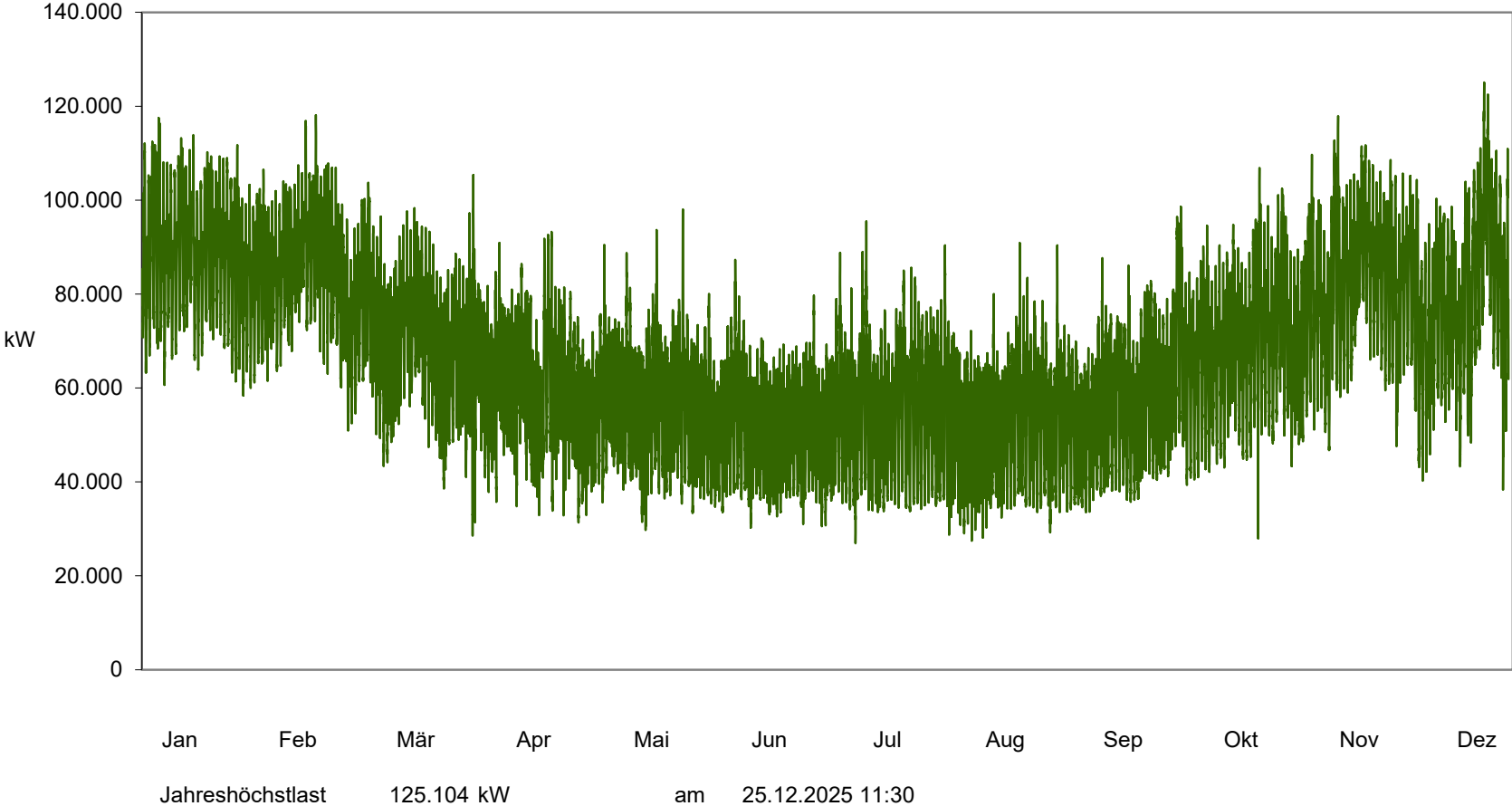
Netzlast 2025 Lastverlauf, Netzebene Niederspannung viertelstündlich
