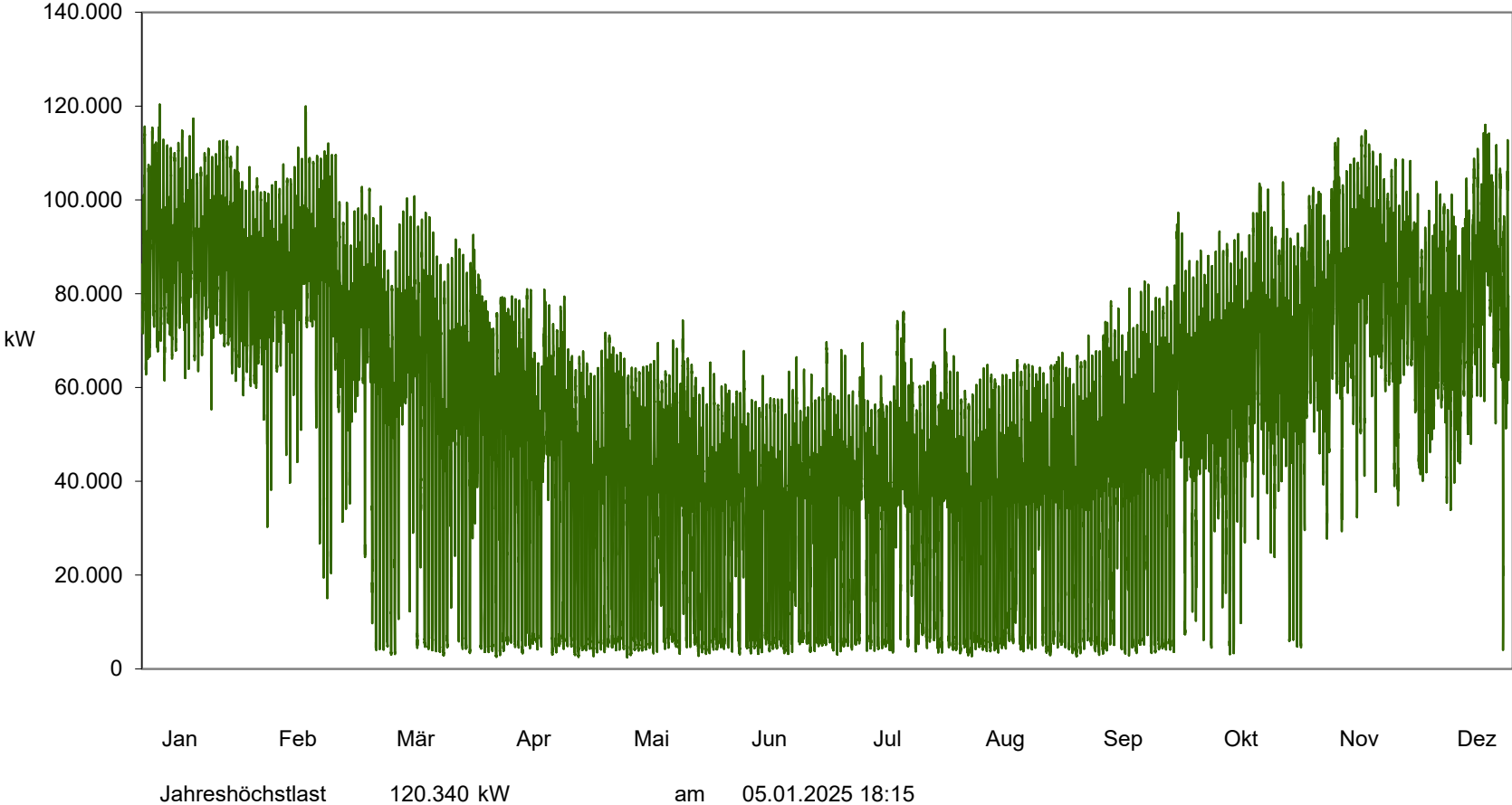
Netzlast 2025 Lastverlauf, Netzebene Mittel-/Niederspannung viertelstündlich
