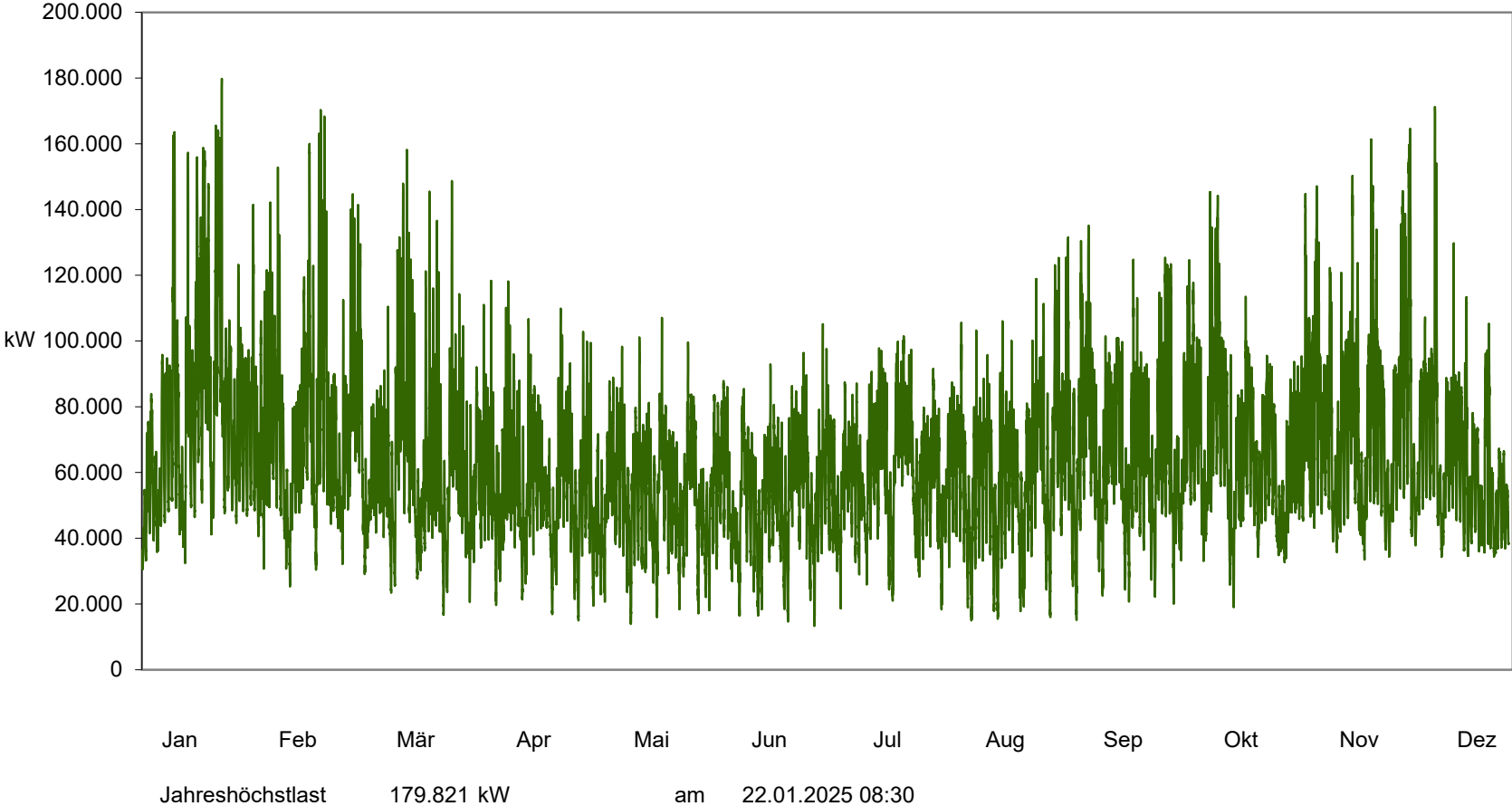
Netzlast 2025 Lastverlauf, Netzebene Hoch-/Mittelspannung viertelstündlich
