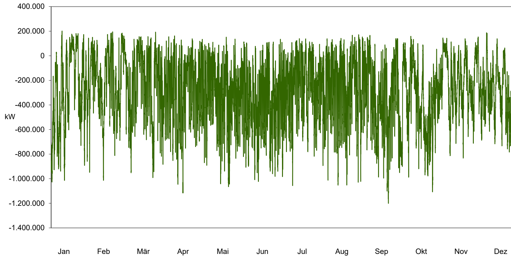
Lastverlauf 2025 Bezug der Hochspannung aus der vorgelagerten Ebene
